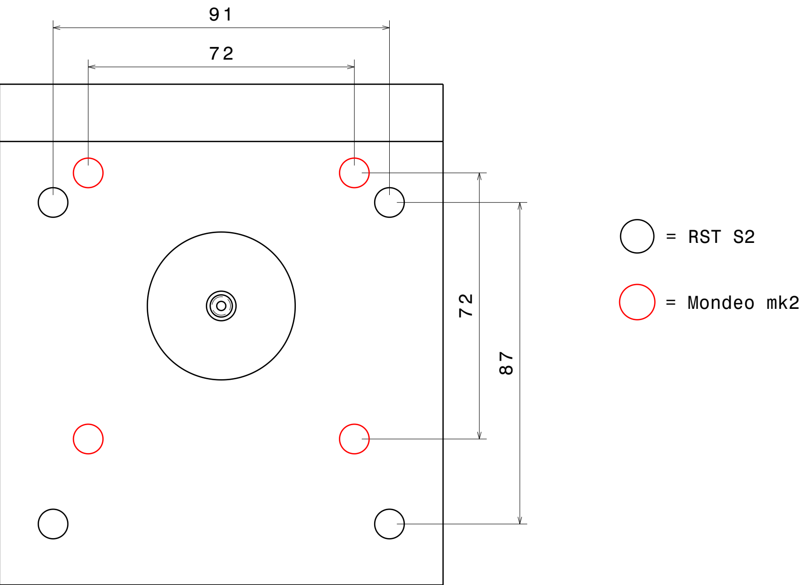
Tehostajat päällekkäin
